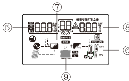
LCD display
